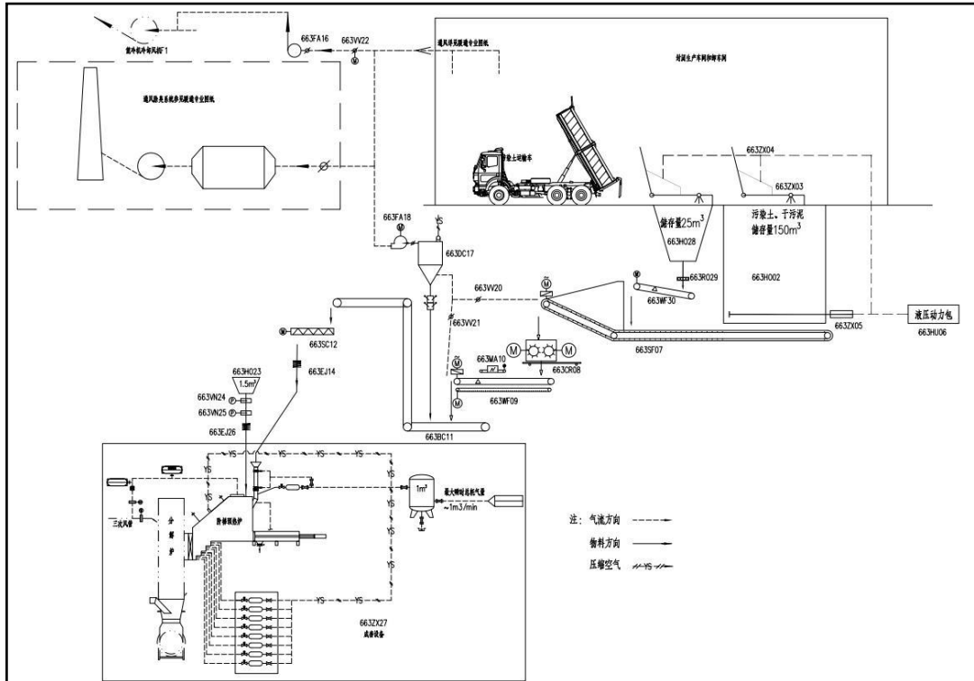
图 2-3 固废(入分解炉)预处理及喂料系统流程图
