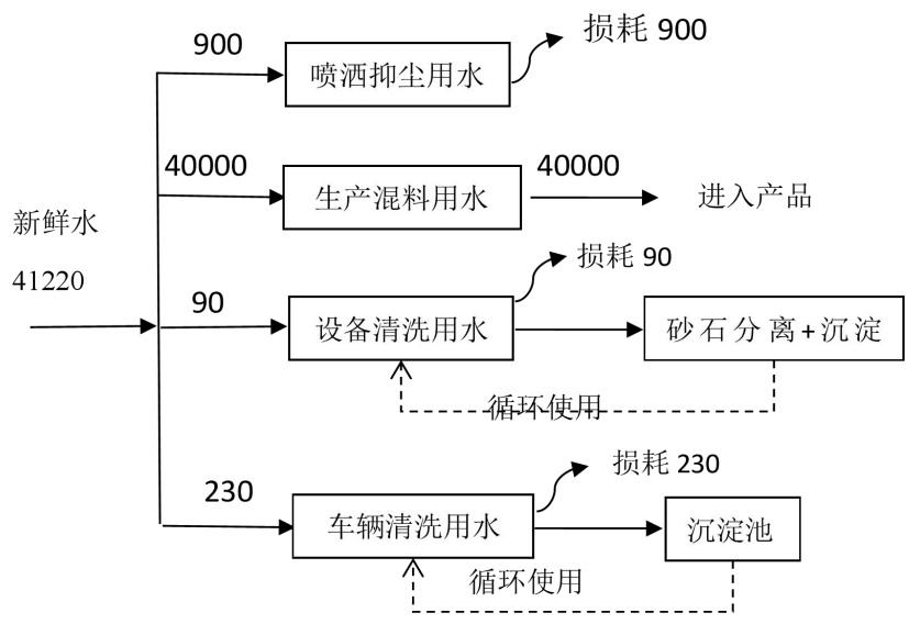
图 2-1 扩建项目水平衡图（单位：m 3 /a）
