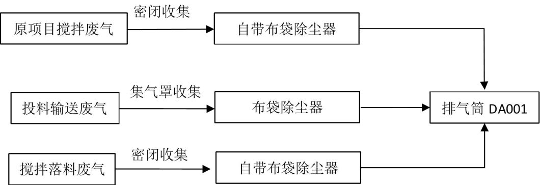
图 4-1 扩建后全厂有组织废气排放流向情况示意图
