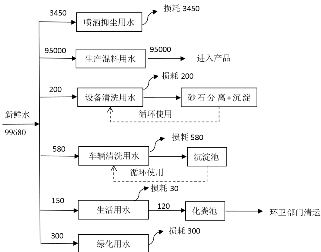
图 2-2 全厂水平衡图 (单位: \text{m}^3/\text{a} )
