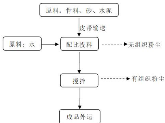
图 2-3 混凝土工艺流程及产污环节图
