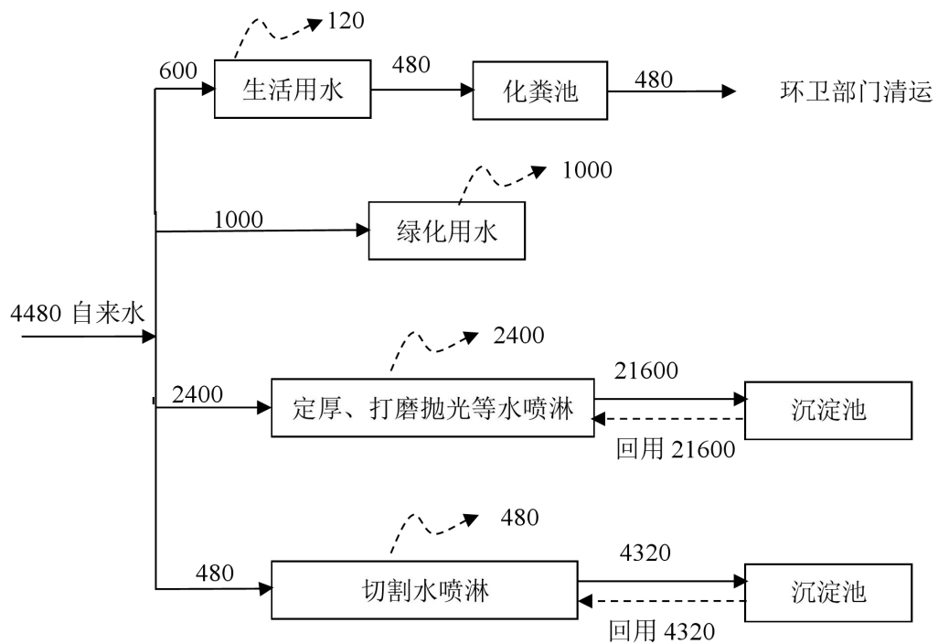
图 2-1 建成后全厂水平衡图 (单位: m³/a)
