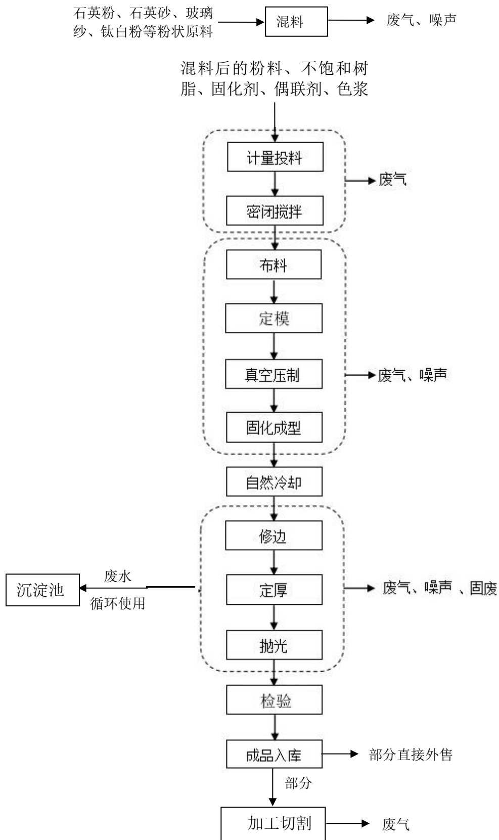
图 2-2 生产工艺流程及排污节点图
