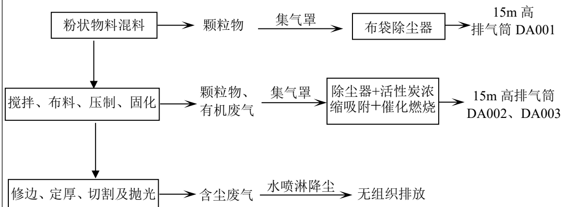
图 2-3 项目废气产生、收集、处理流程图
