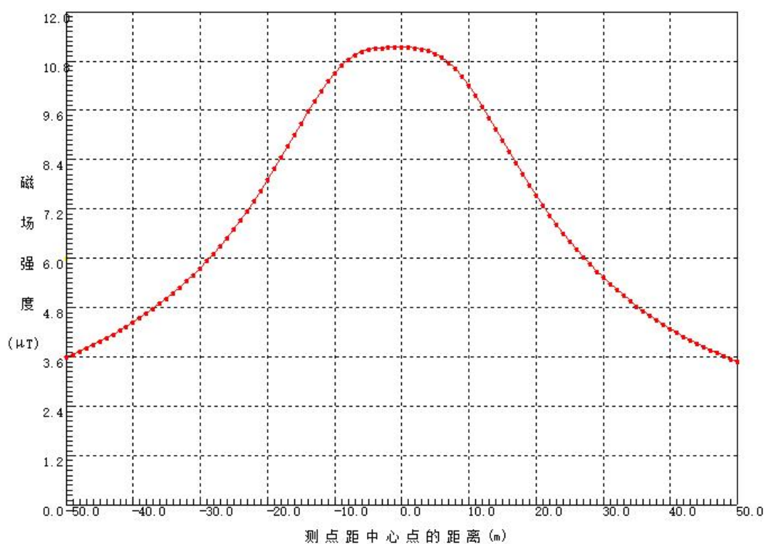
图 7 源邵线架空线路（单回单挂）工频磁感应强度趋势图
