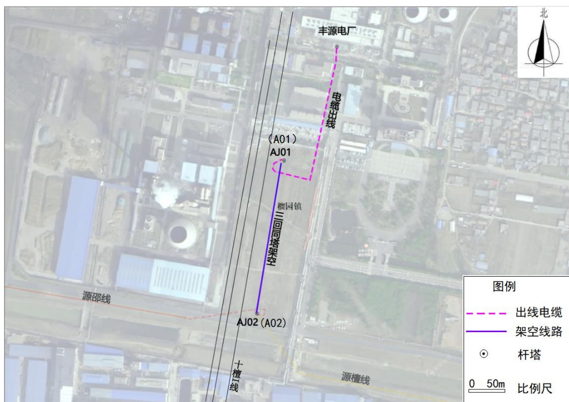
图 2-7 出线走廊示意图
