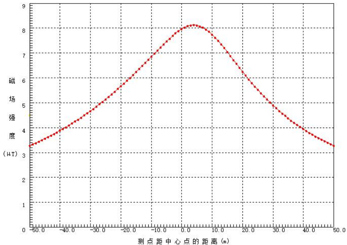
图3 A01至A02架空线路（三回双挂）工频磁感应强度趋势图
