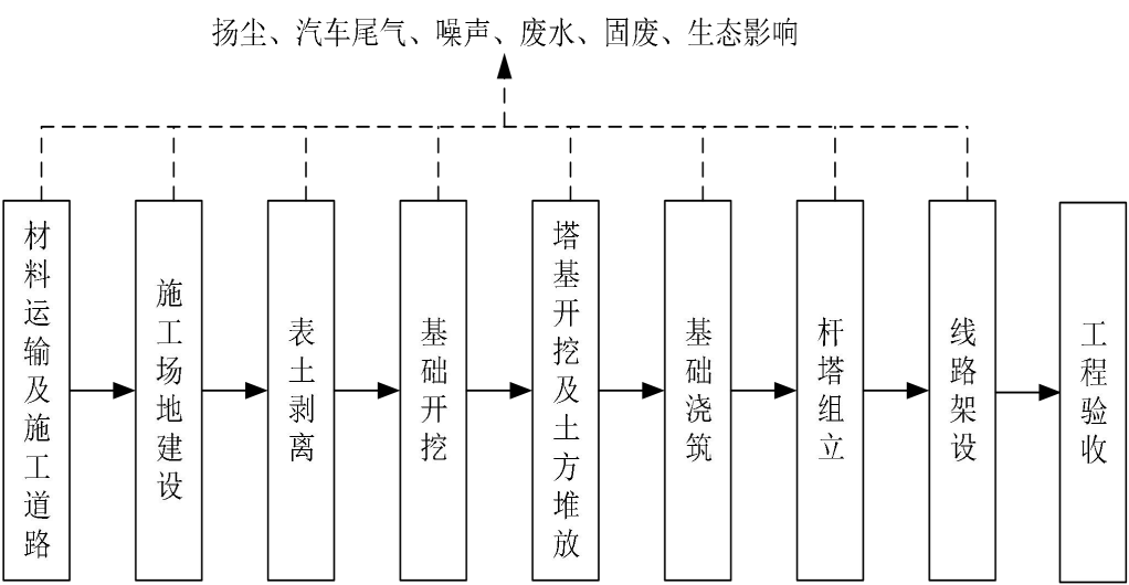
图 2-4 架空输电线路施工工艺流程示意图
