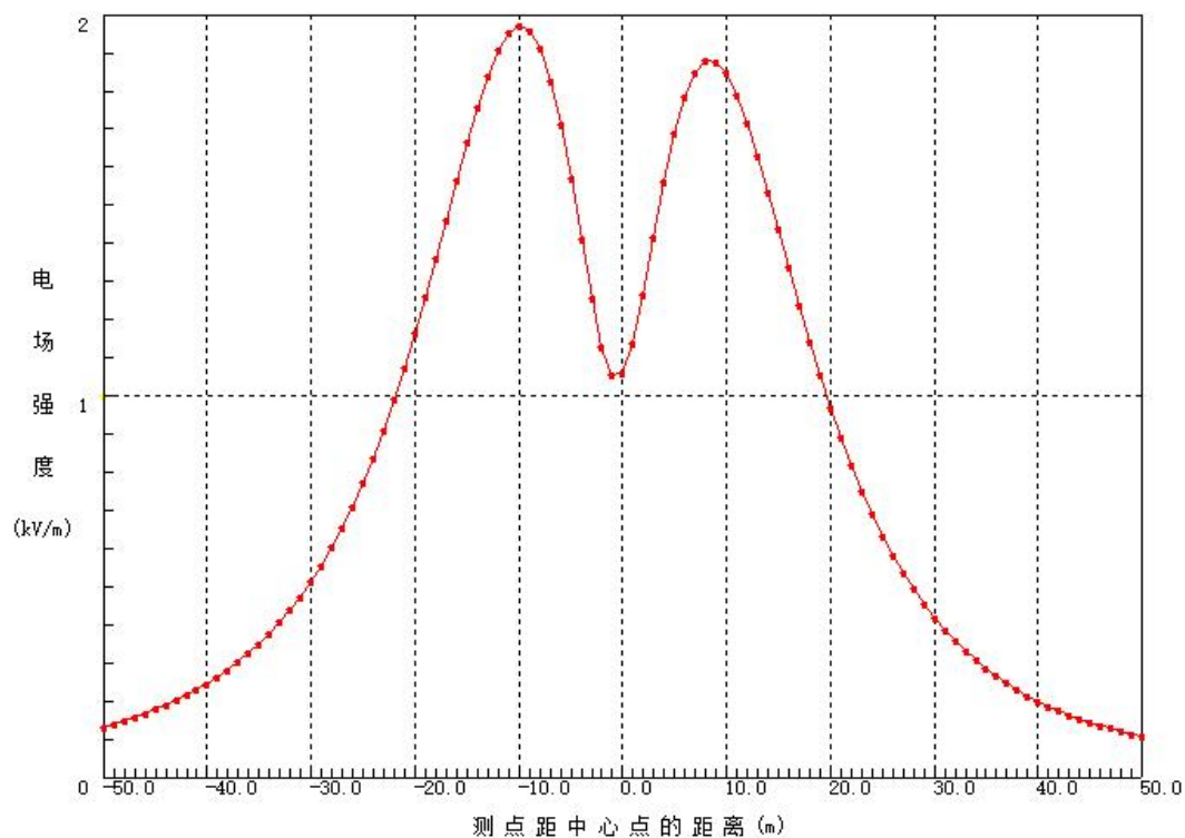
图 6 源邵线架空线路（单回单挂）工频电场强度趋势图
