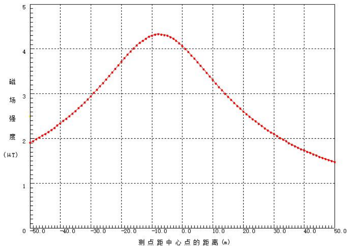
图 5 源檀线架空线路（双回单挂）工频磁感应强度趋势图
