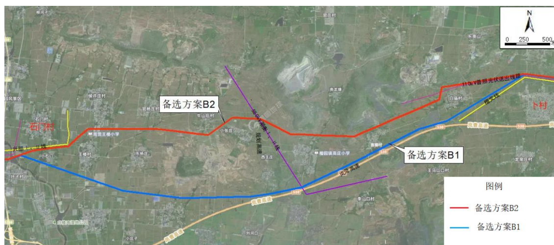
图 2-22 备选方案 B 在卜村~石门村段与电力线路穿越情况
