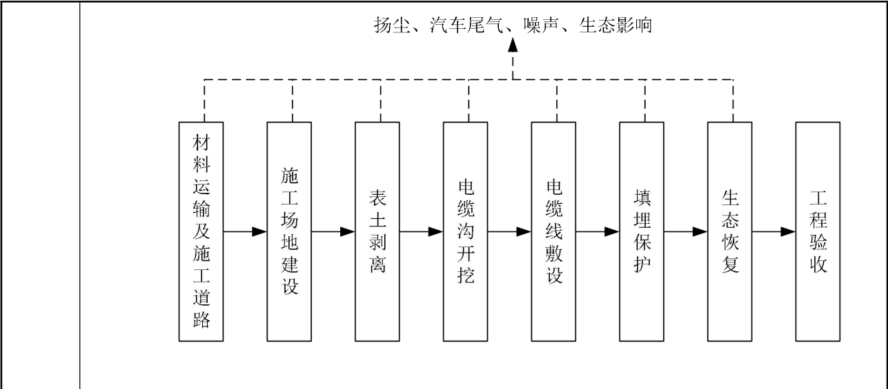
图 2-5 电缆线路施工工艺流程示意图
