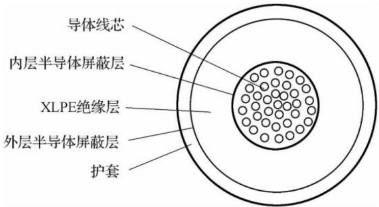
图 8 电缆结构及断面示例
