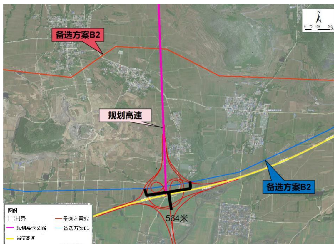
图 2-20 备选方案 B 与规划高速公路跨越关系示意图
