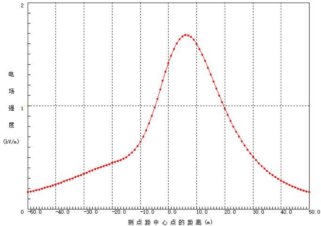
图2 A01至A02架空线路（三回双挂）工频电场强度趋势图
