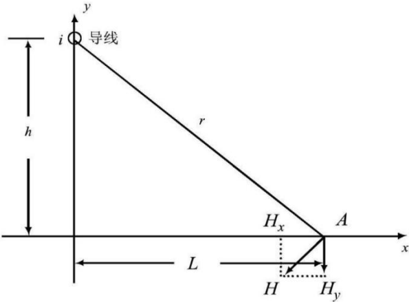
图 1 磁场向量图
