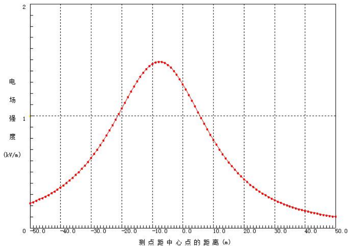
图 4 源檀线架空线路（双回单挂）工频电场强度趋势图
