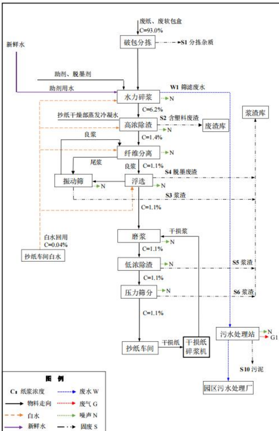
图 2.6-1 脱墨浆生产工艺流程及产排污节点图
