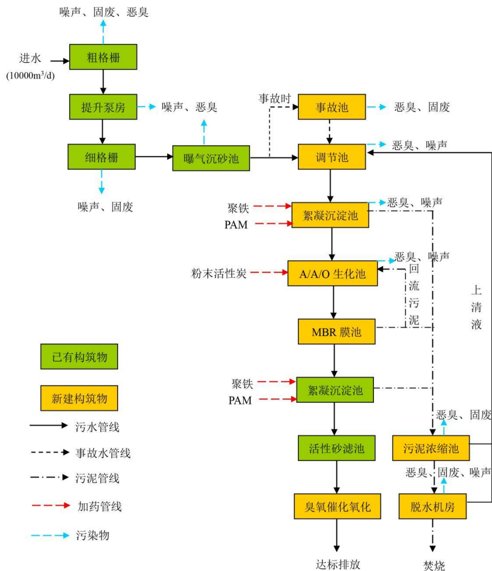
图 4.3-1 滕州市级索镇污水处理厂改造后工艺流程图
