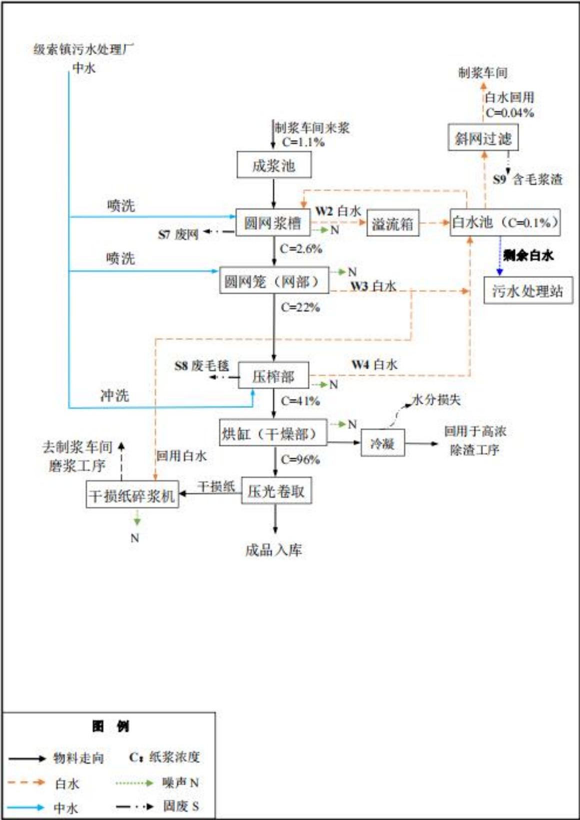
图 2.6-2 抄纸生产工艺流程及产排污节点图
