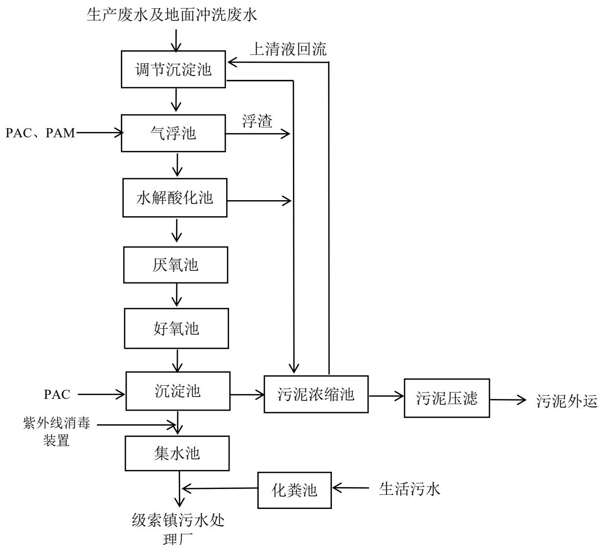
图 2.9-1 污水处理站污水处理工艺流程图
