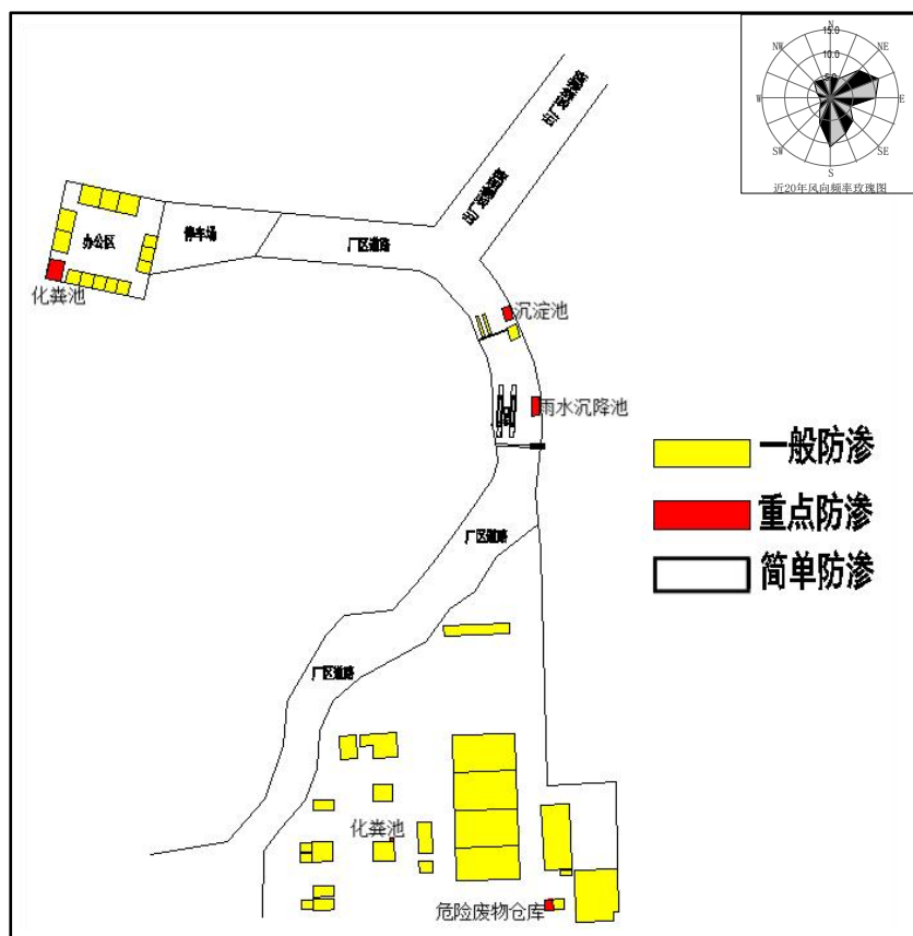
图6.3-1 建设项目分区防渗图
