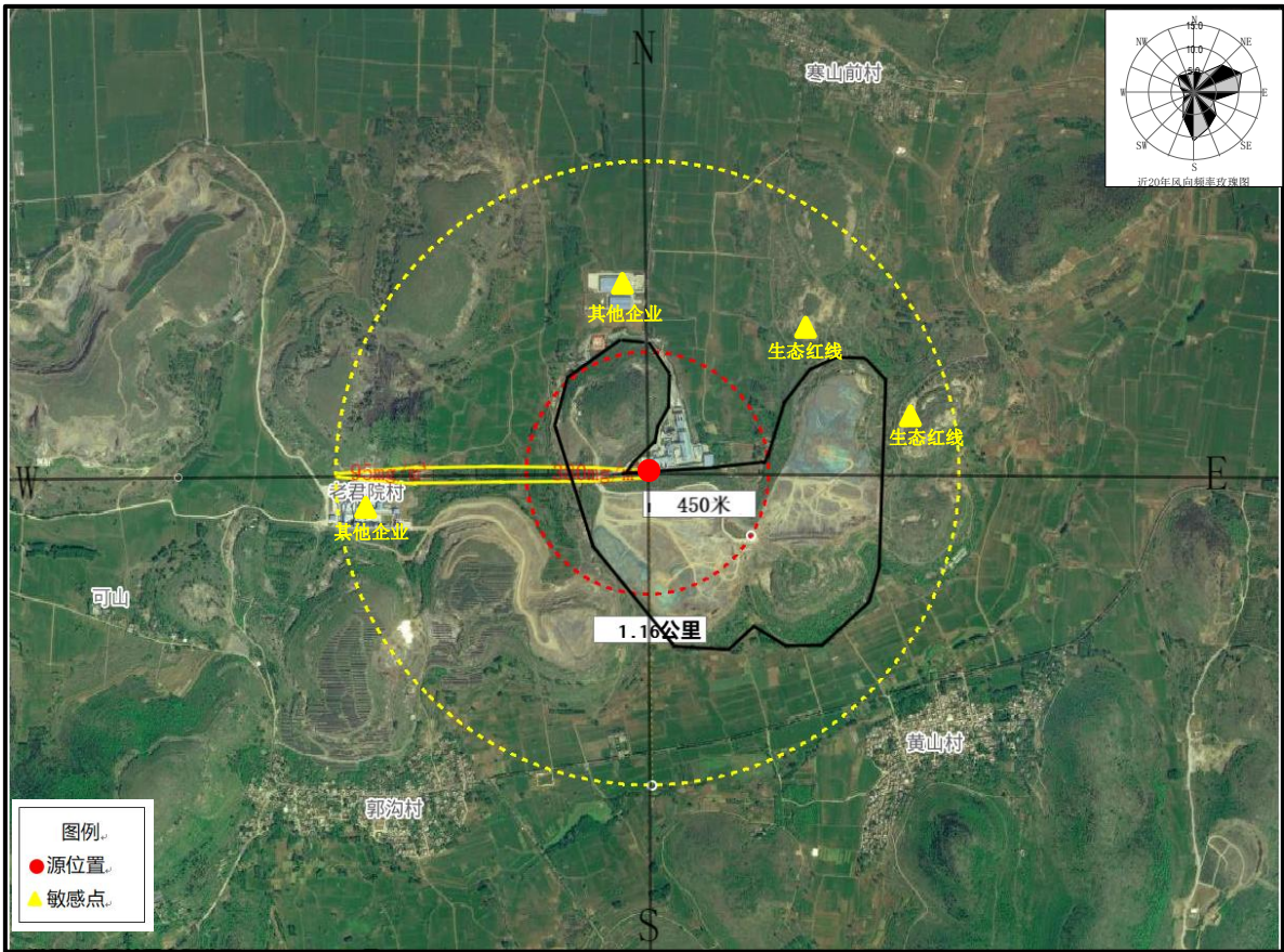
图7.7-1 最不利气象条件下CO最大影响范围图
