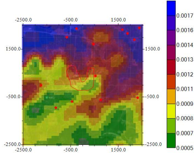
图6.1-4 本项目区域网格点PM 10 最大日均地面浓度贡献等值线图
