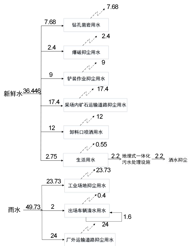
图2.1-1 现有项目水平衡图 (m³/d)
