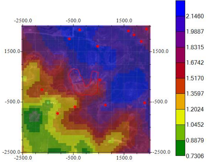
图6.1-8 非正常工况下PM 10 最大浓度贡献等值线图
