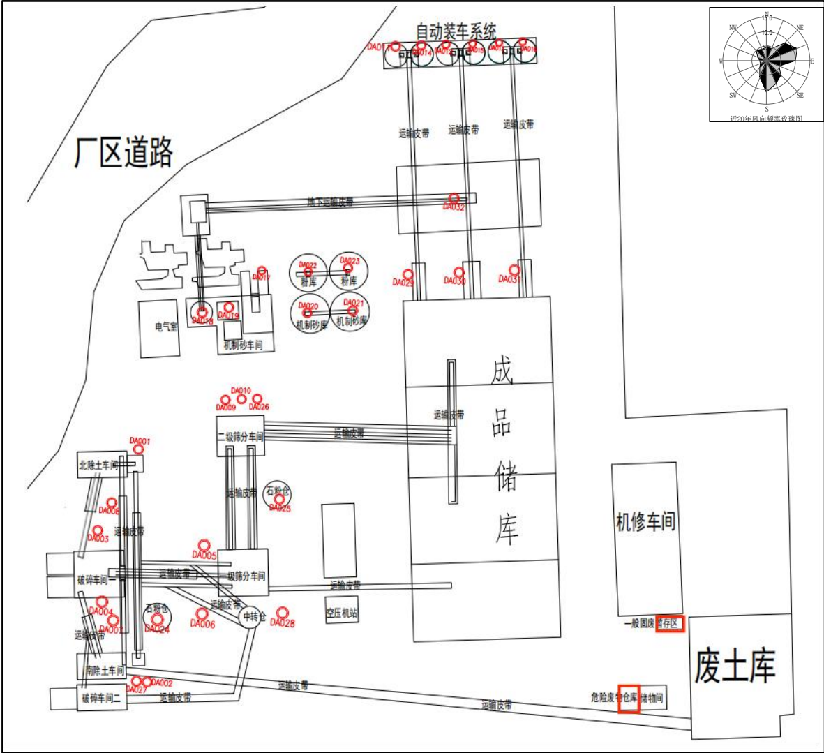
图2.1-4 现有工程生产区环保设施布置图
