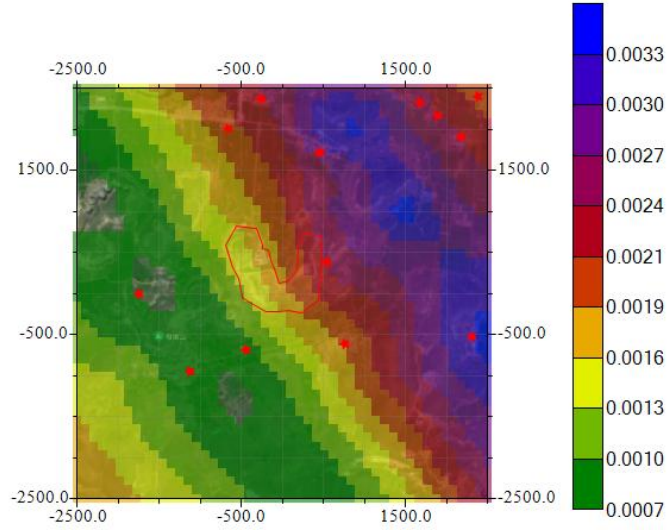
图6.1-5 本项目区域网格点TSP最大日均地面浓度贡献等值线图
