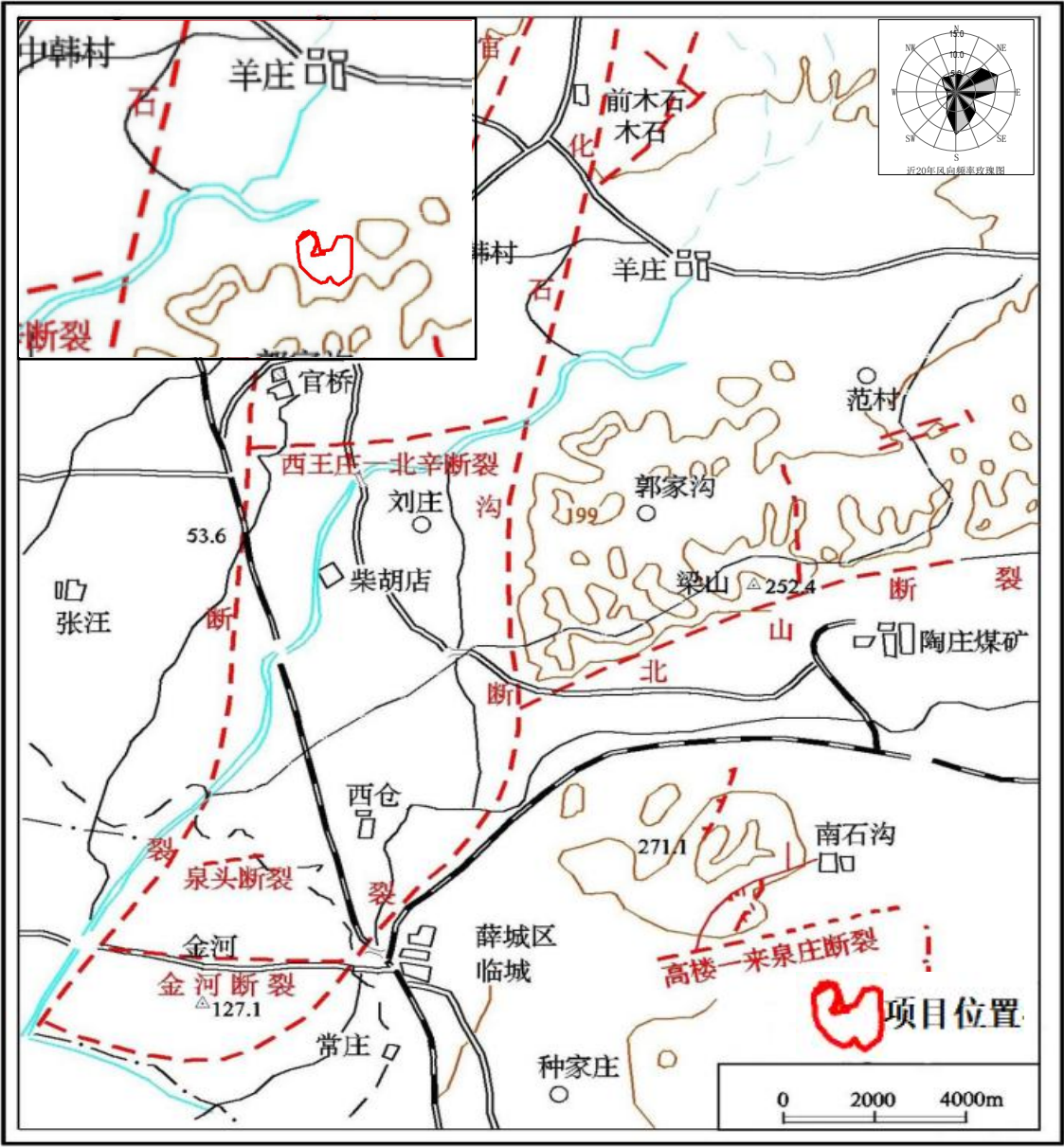
图4.1-5 区域构造略图
