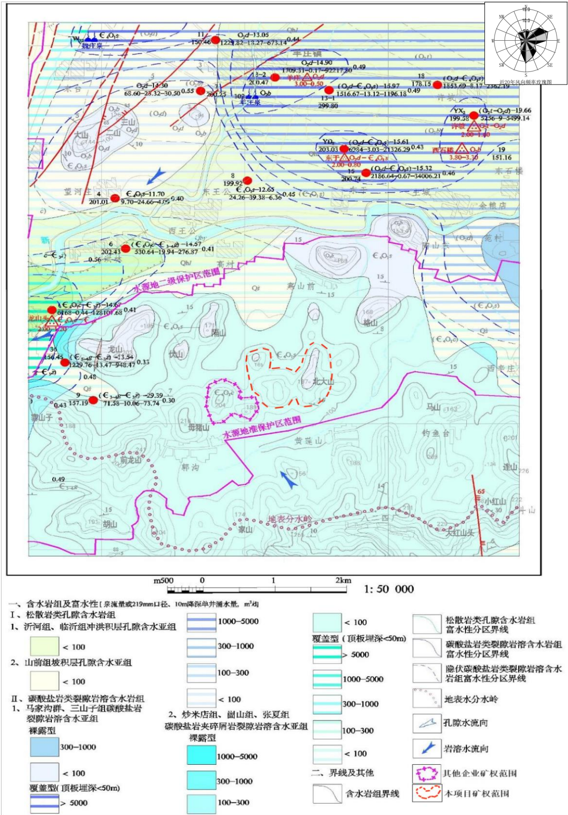
图4.1-7 项目与区域水文地质关系图
