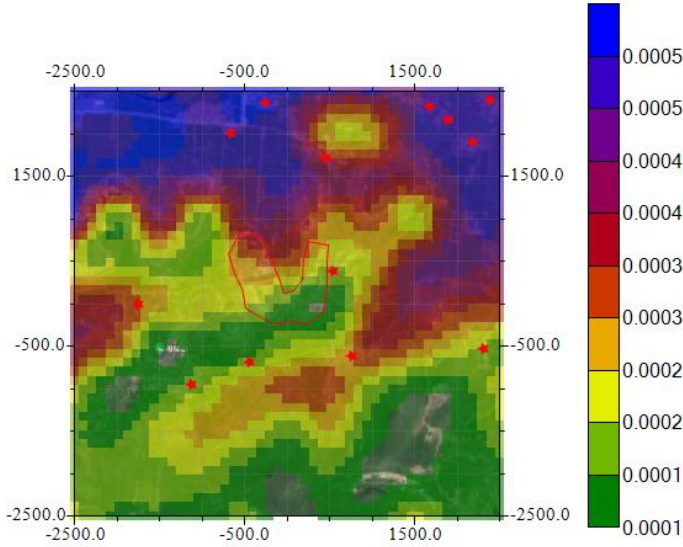
图6.1-6 本项目区域网格点PM 10 最大年均地面浓度贡献等值线图
