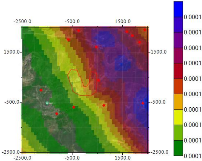
图6.1-7 本项目区域网格点TSP最大年均地面浓度贡献等值线图
