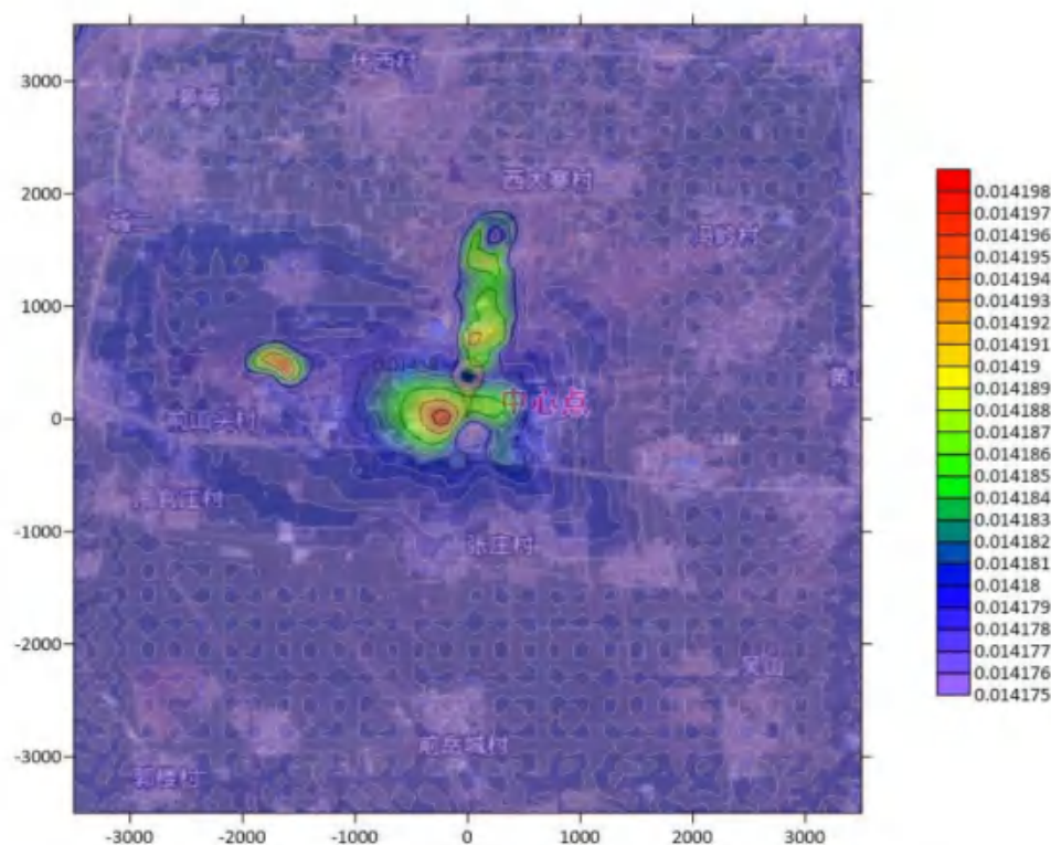
图 4.1-33 考虑在建源并叠加现状后区域格点 \text{SO}_2 年均浓度分布图
