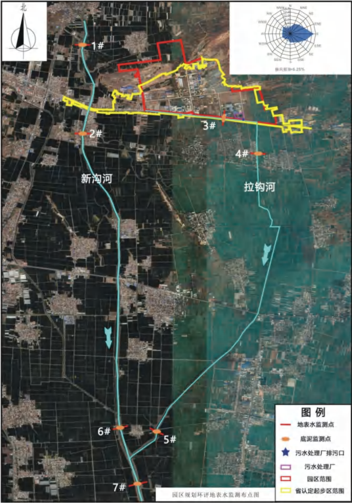
图 3.3-2 园区规划环评地表水监测布点图
