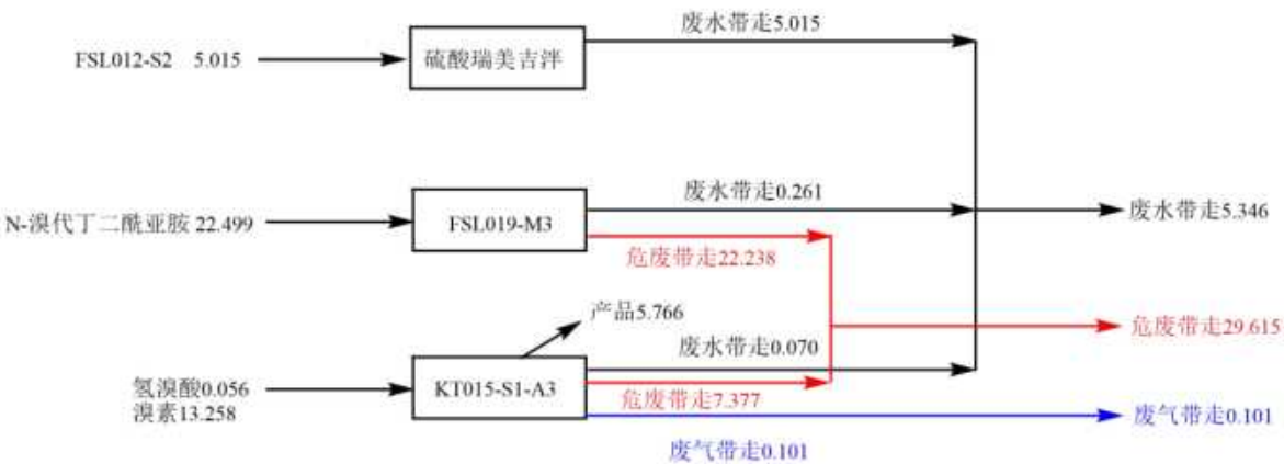
图 2.17-9 拟建项目溴平衡图（单位： t/a）
