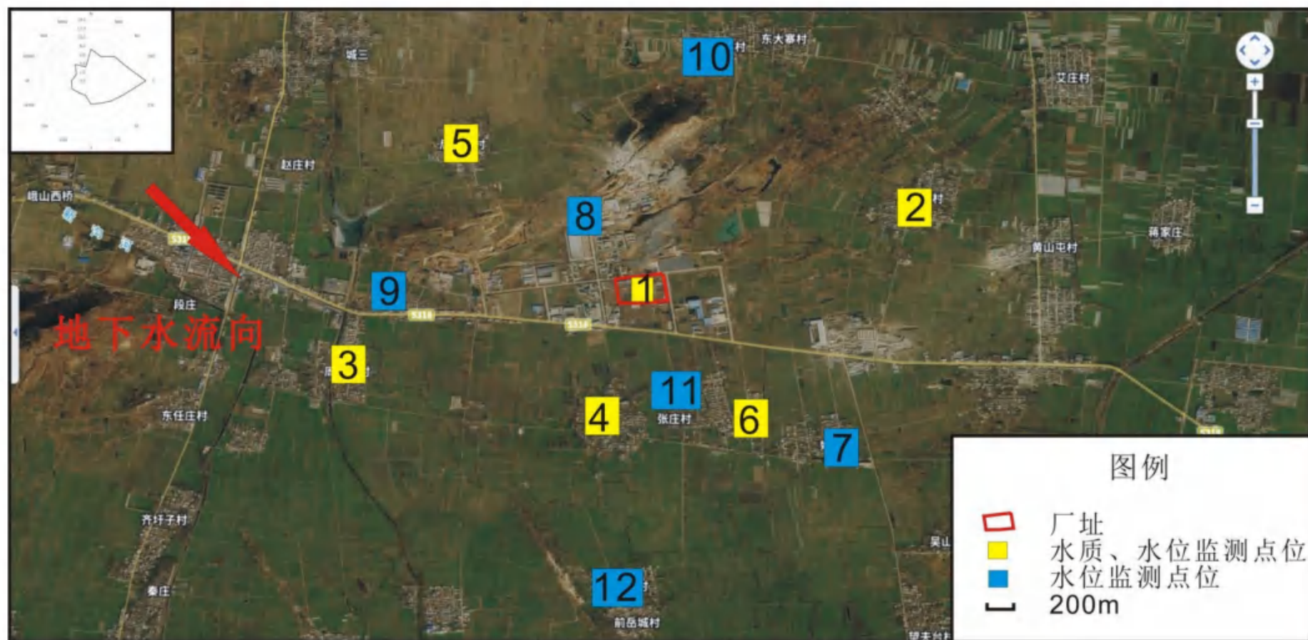
图 3.4-1 拟建项目地下水监测布点图
