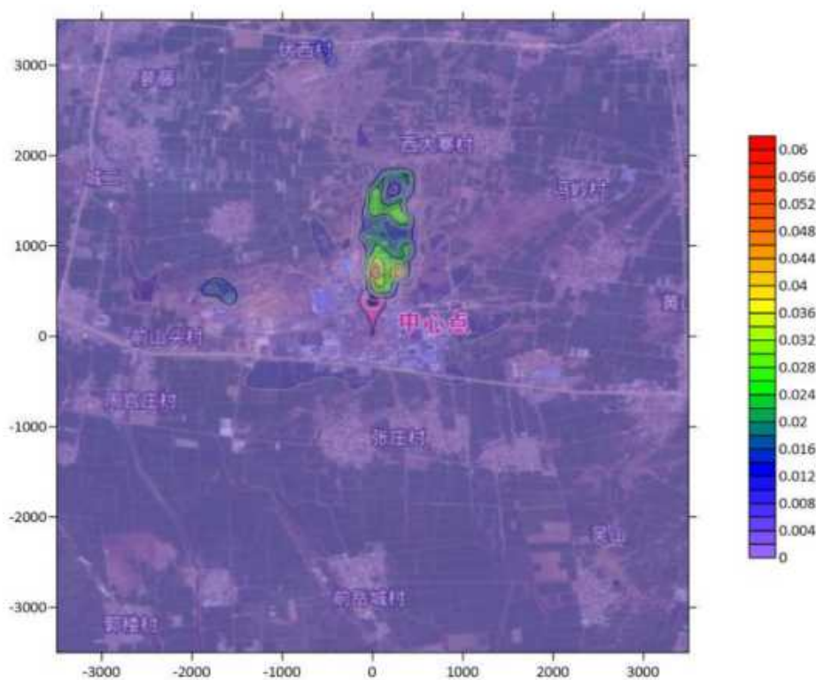
图 4.1-6 拟建项目区域格点 \text{NO}_2 最大小时地面浓度贡献值浓度分布图
