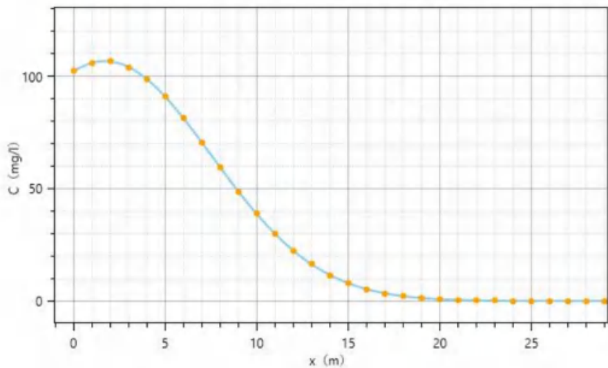
图 5.7-4a 1000d 污染物浓度预测结果
