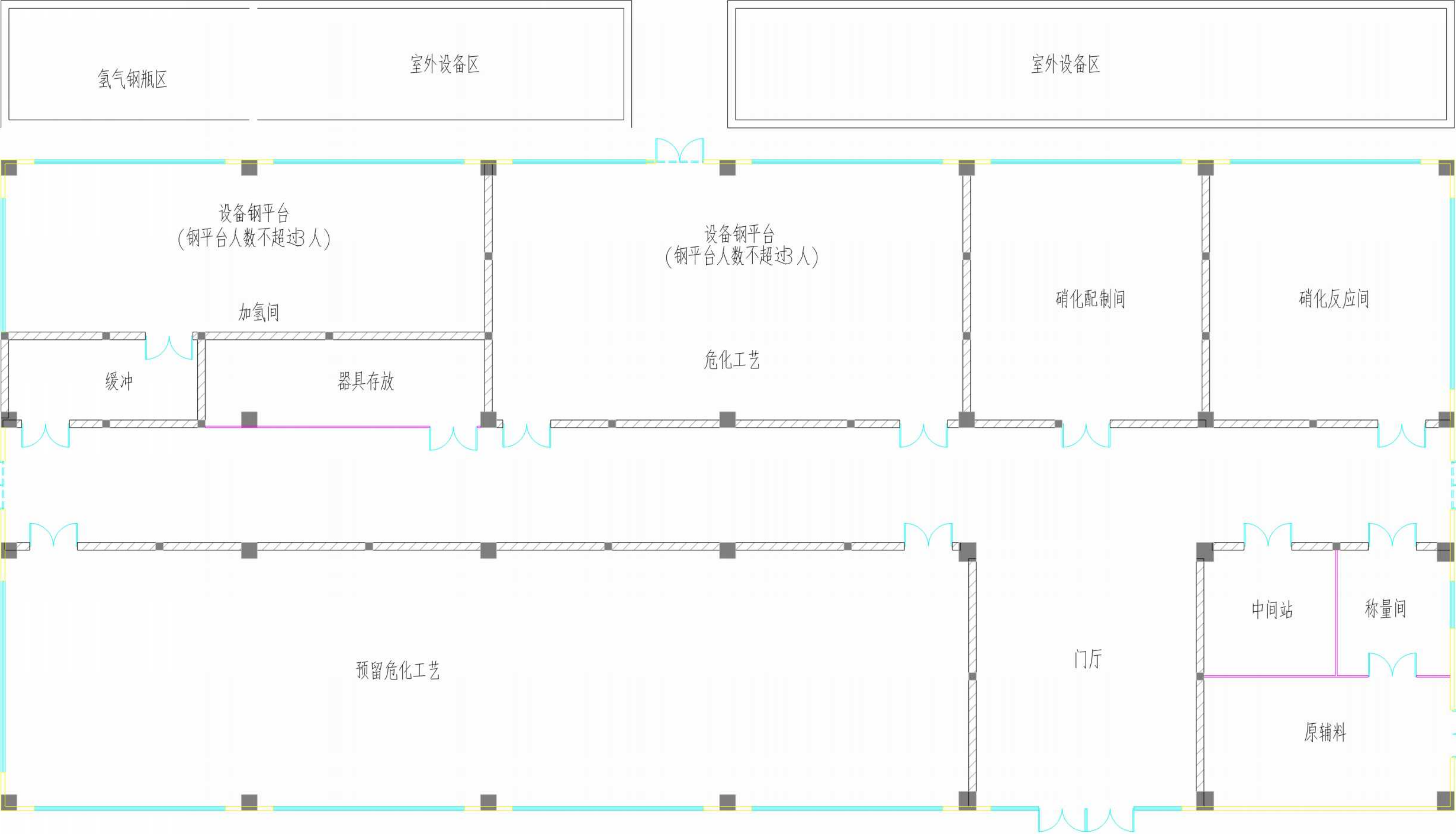
一层平面图
