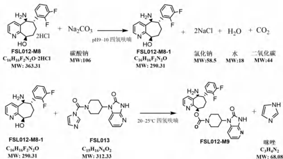
图 2.5-11 缩合反应式
