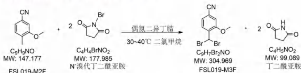
图 2.12-6 FSL019-M3F 制备反应式
