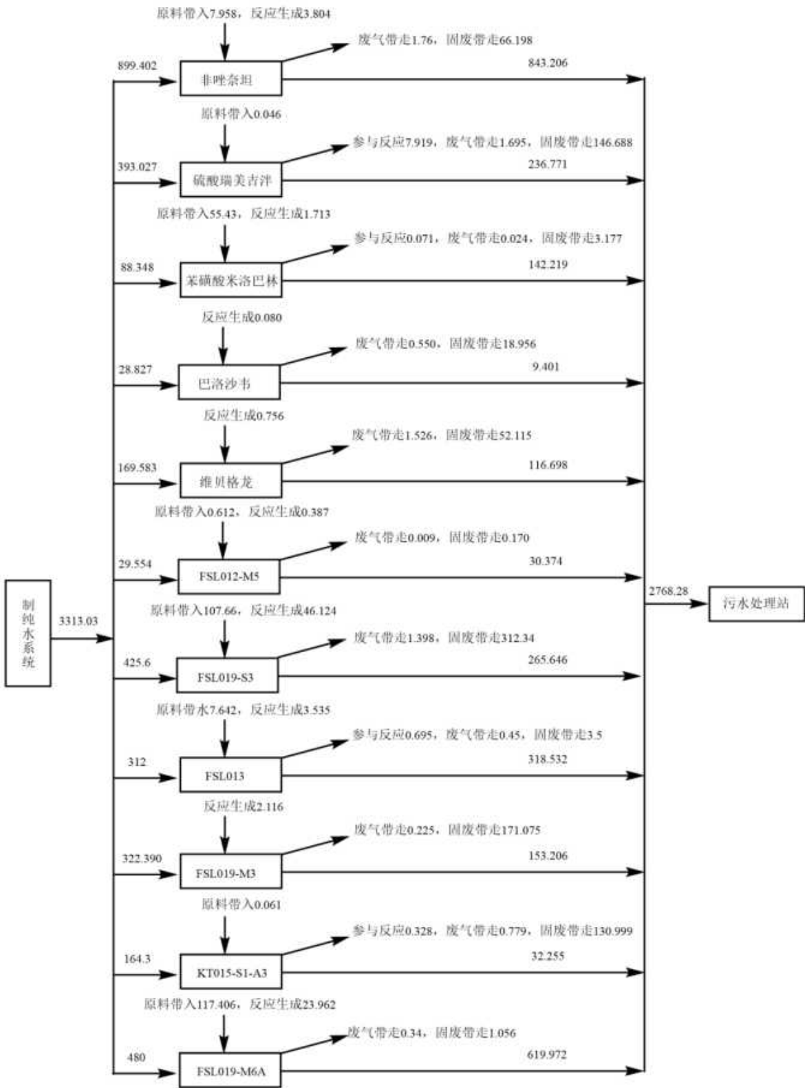
图 2.18-3 拟建项目工艺水平衡（单位：m³/a）
