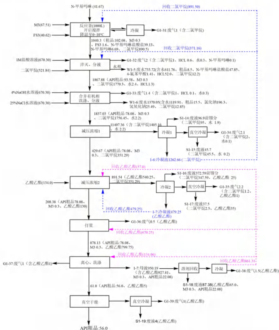
图 2.4-18 非唑奈坦 API 粗品合成物料平衡图 (单位: kg/批次)
