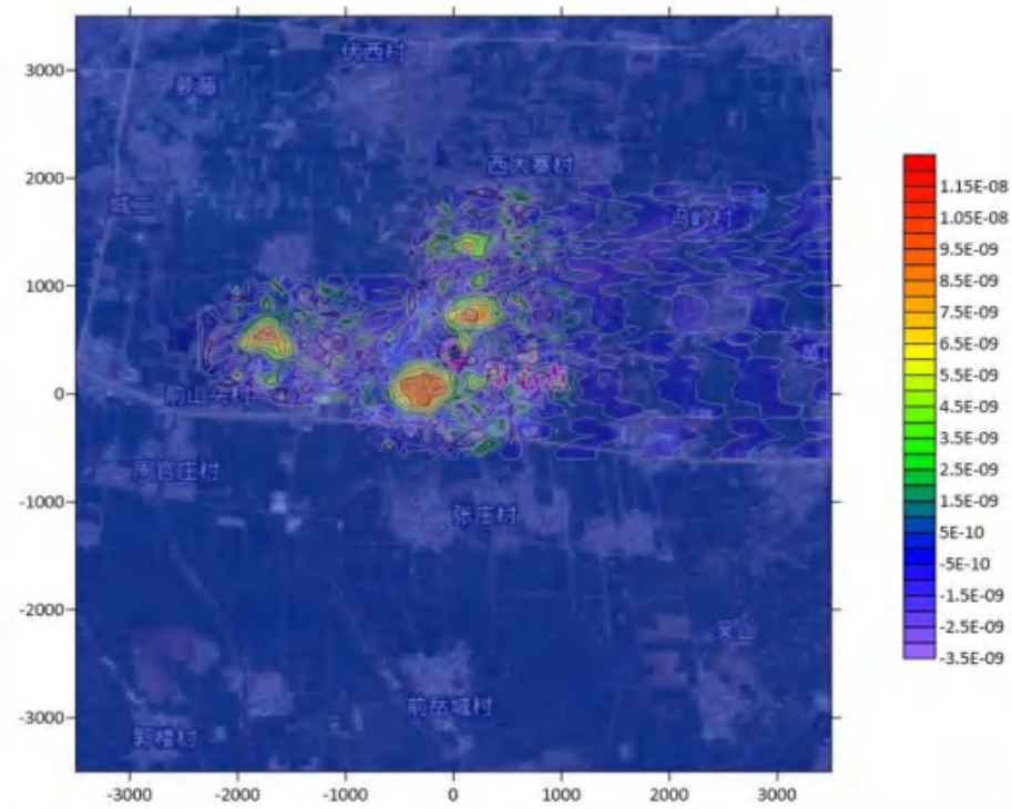
图 4.1-31 拟建项目区域格点二噁英年均地面浓度贡献值浓度分布图 (注：二噁英的单位为 \text{ng}/\text{m}^3 )
