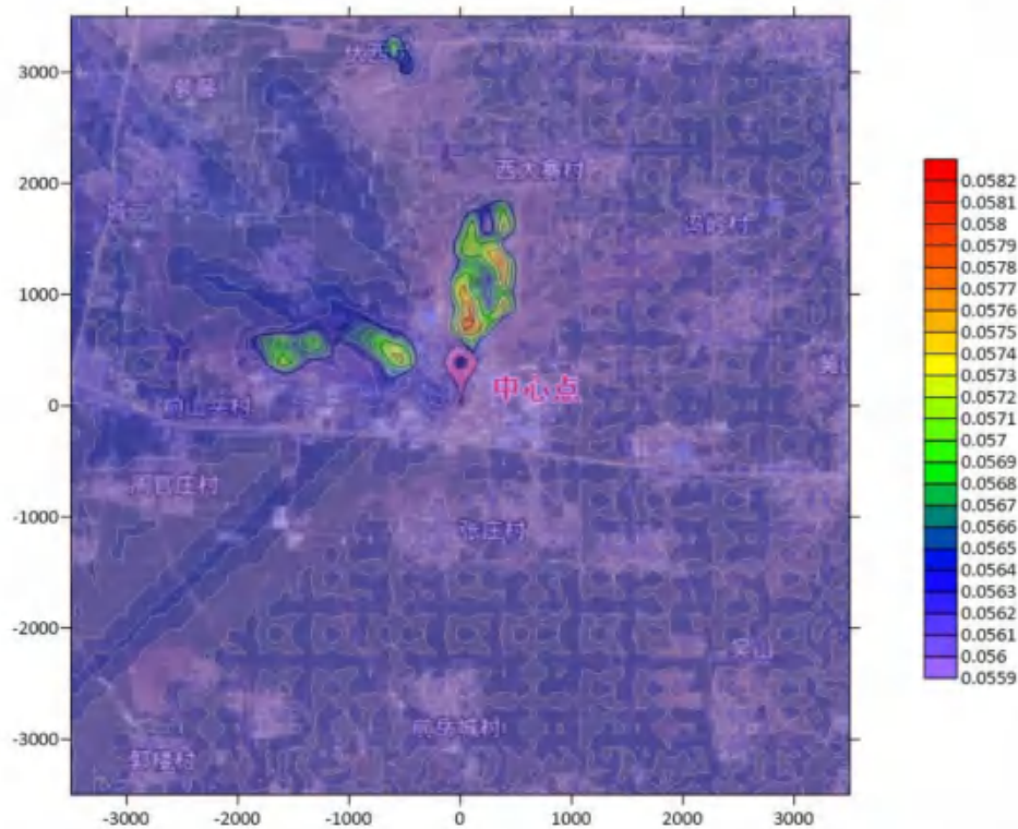
图 4.1-34 考虑在建源并叠加现状后区域格点 \text{NO}_2 最大保证率日均浓度分布图
