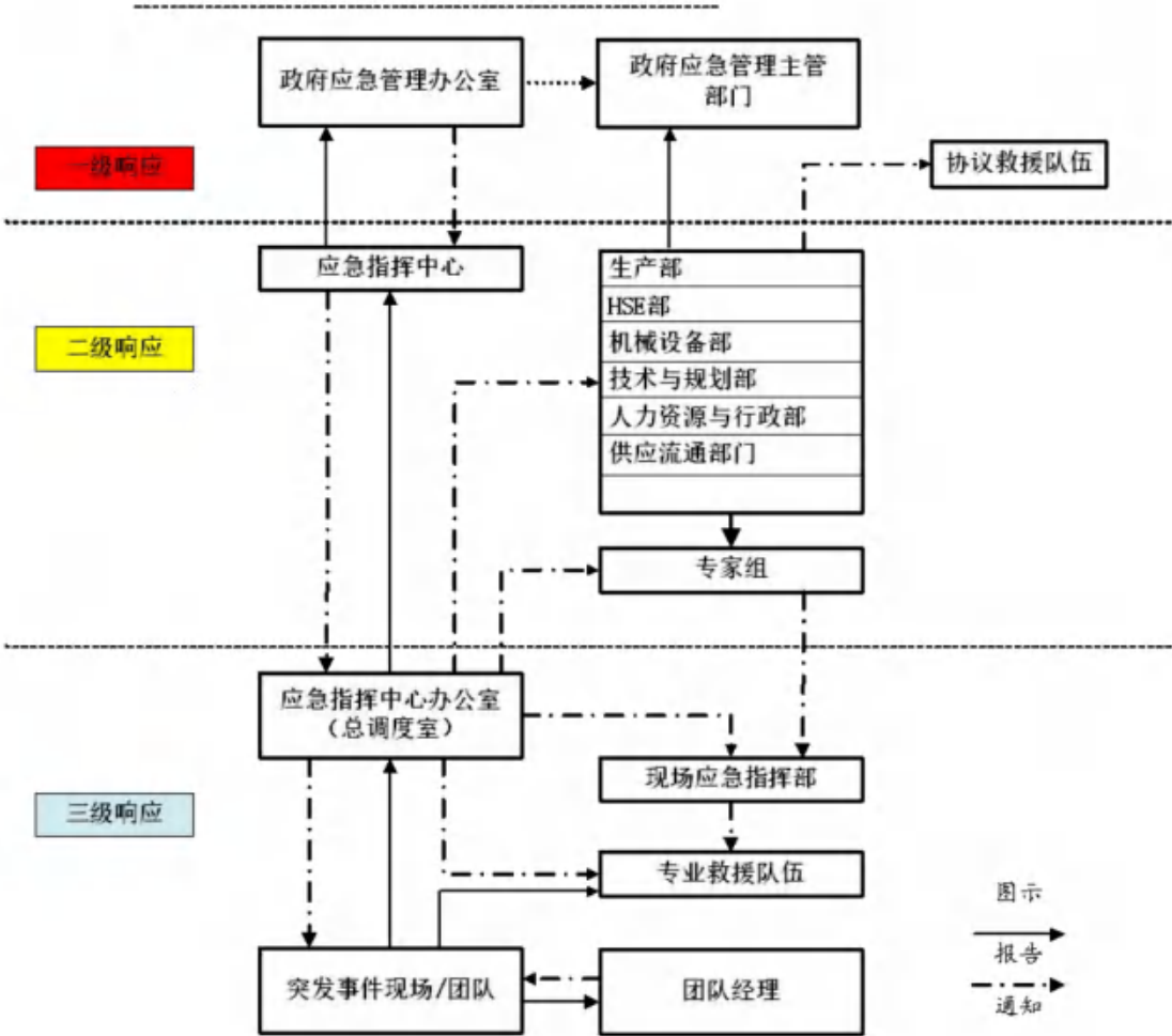
图 5.11-2 应急报告流程示意图
