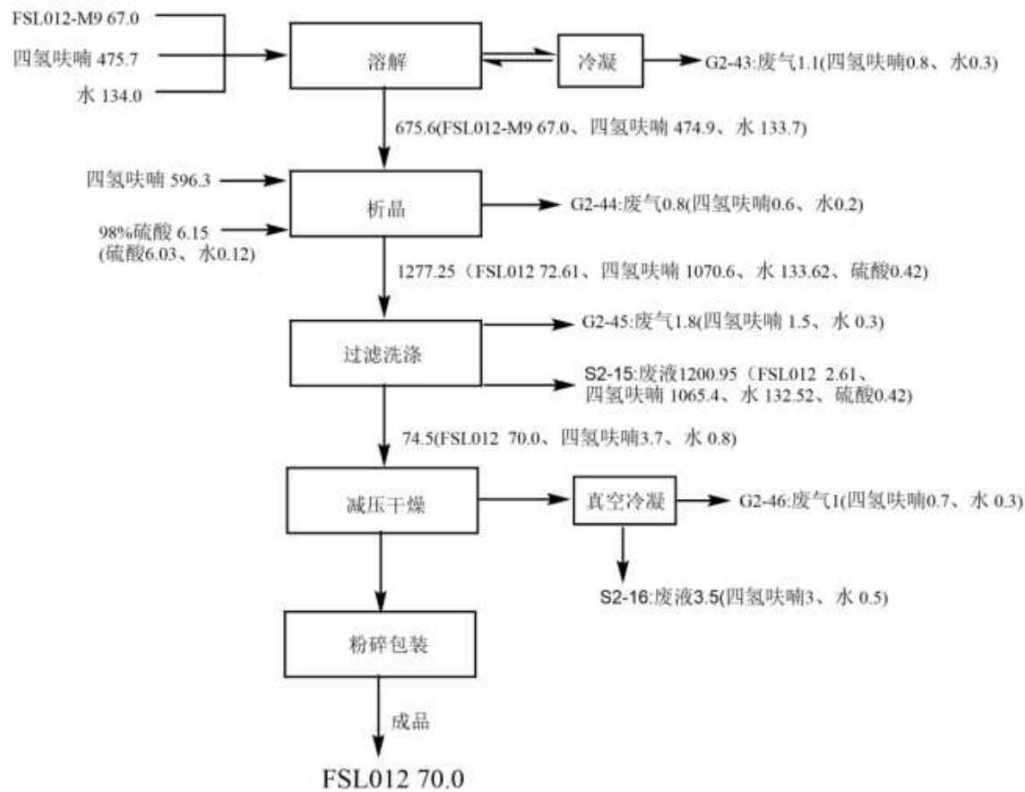
图 2.5-16 硫酸瑞美吉洋 FSL012 物料平衡图（单位：kg/批次）
