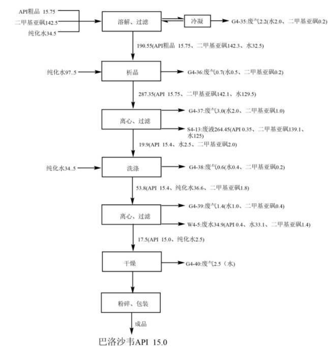
图 2.7-16 巴洛沙韦 API 精制物料平衡图（单位：kg/批次）
