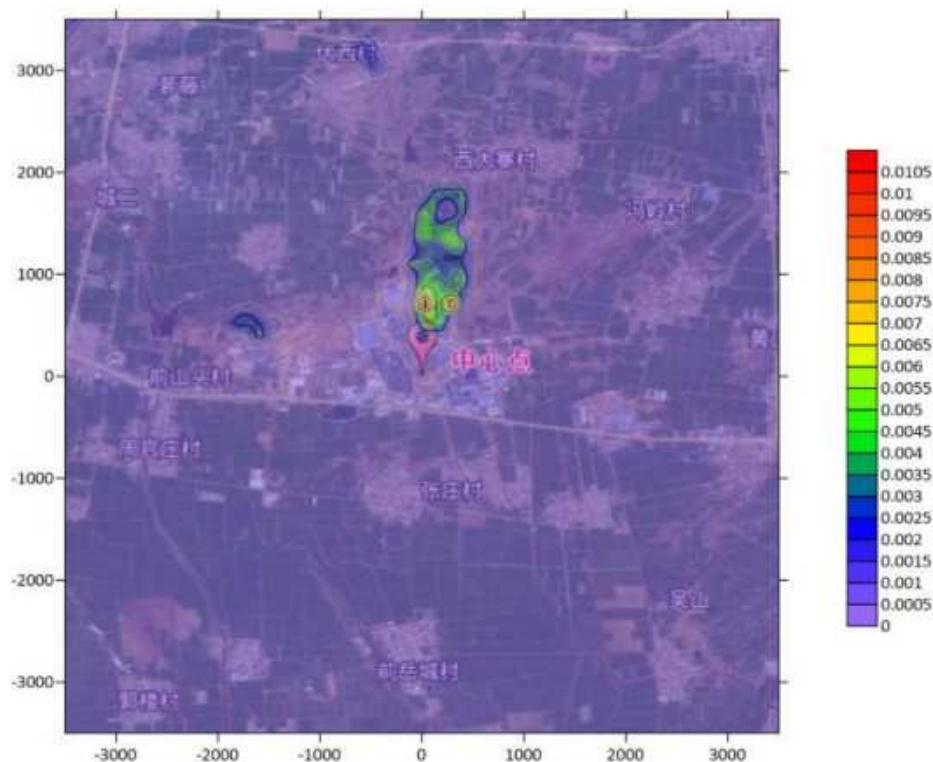
图 4.1-3 拟建项目区域格点 \text{SO}_2 最大小时地面浓度贡献值浓度分布图
