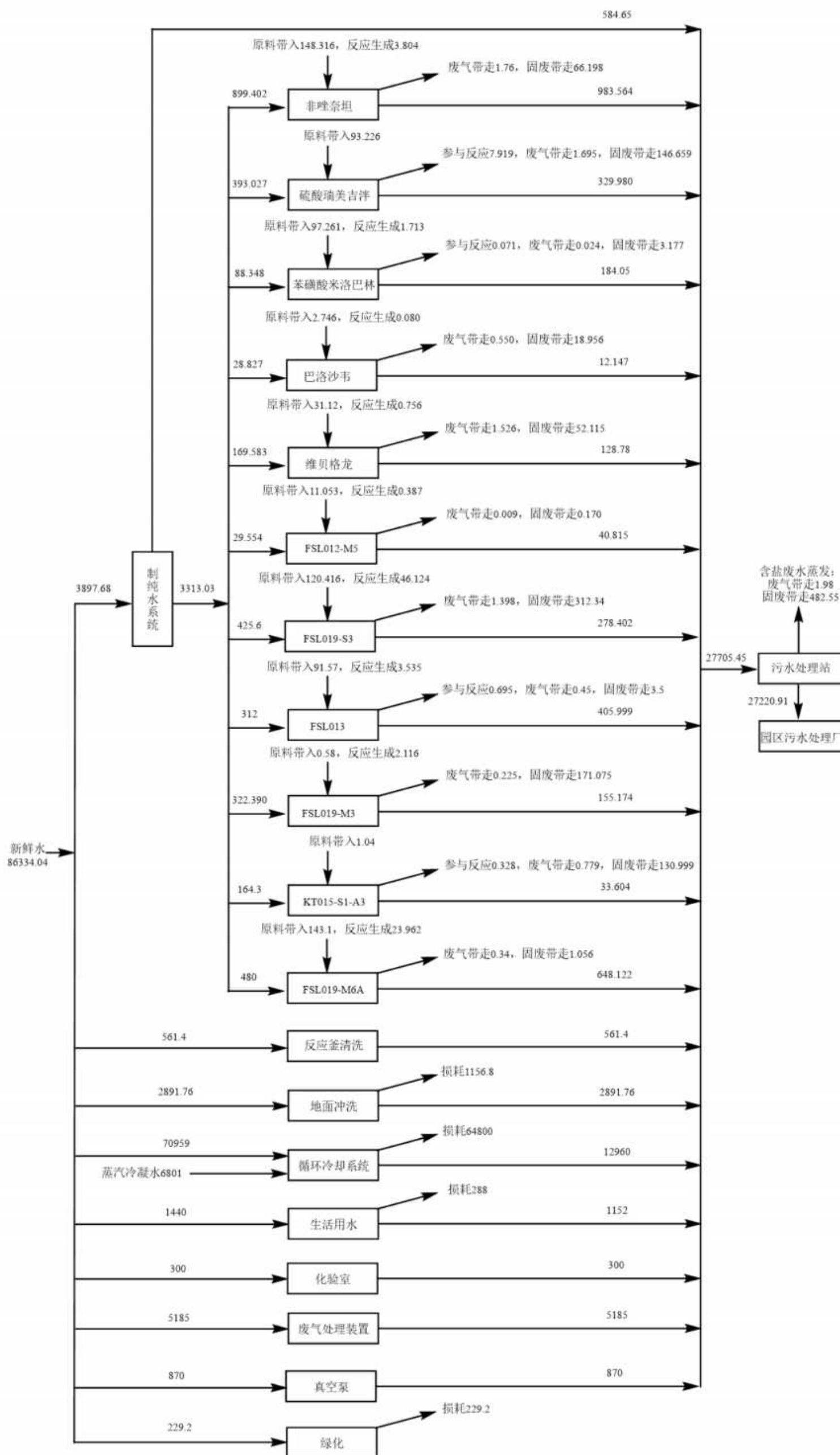
图 2.18-4 拟建工程全厂水平衡图 (单位: \text{m}^3/\text{a} )
