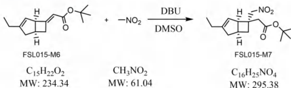
图 2.6-8 加成反应式
