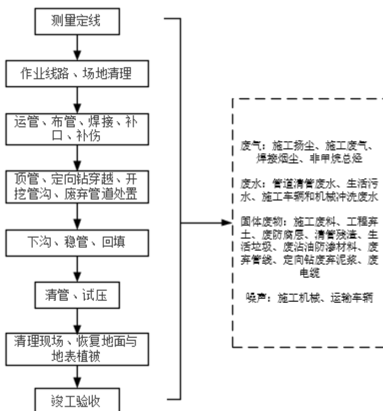
图 2.10-1 管道工程主要施工过程
