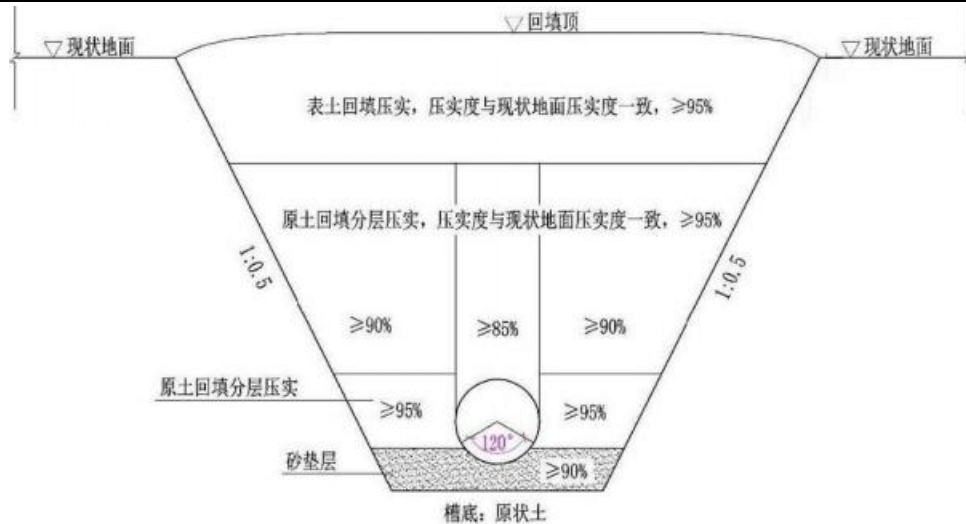
图 5.7-1 土壤保护措施示意图
