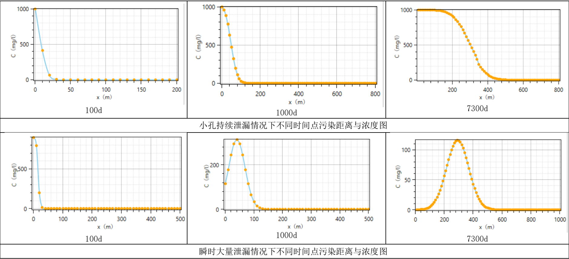
图 5.3-2 管线泄漏对地下水影响预测结果图
