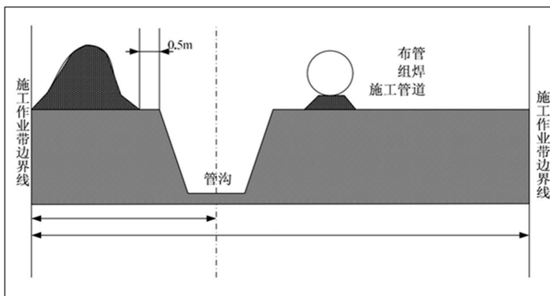
图 2.10-2 开挖施工断面示意图
