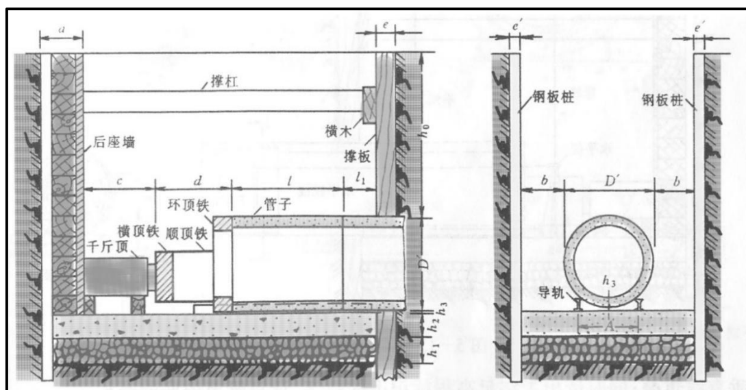
图 2.10-3 顶管施工工作坑构造和设施示意图
