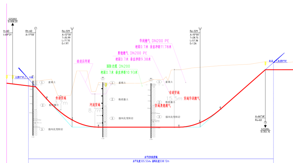
图 2.4-5 定向钻穿越燃气管道剖面图
