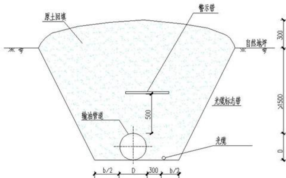
图 2.4-3 管道敷设典型图
