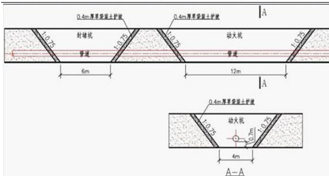
图 2.10-13 封堵连头作业坑示意图
