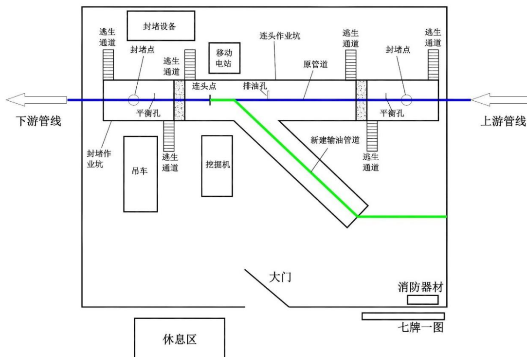
图 2.10-12 旧管道处置施工平面布置示意图
