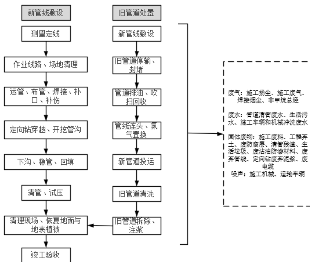
图 2.10-16 管道施工工艺流程图
