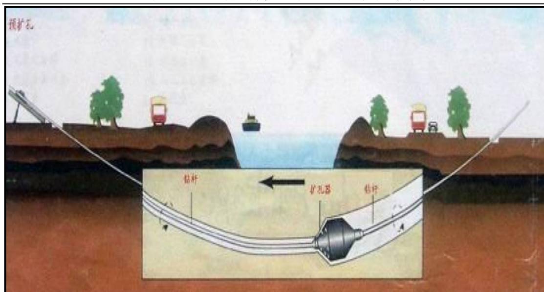
图 2.10-6 定向钻穿越施工预扩孔过程断面示意图
