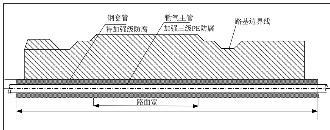
图 2.10-4 公路穿越施工方式断面示意图
