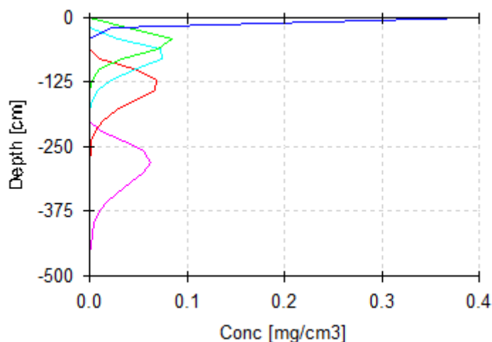
图 5.6-3 不同时刻石油类浓度-剖面深度变化曲线图
