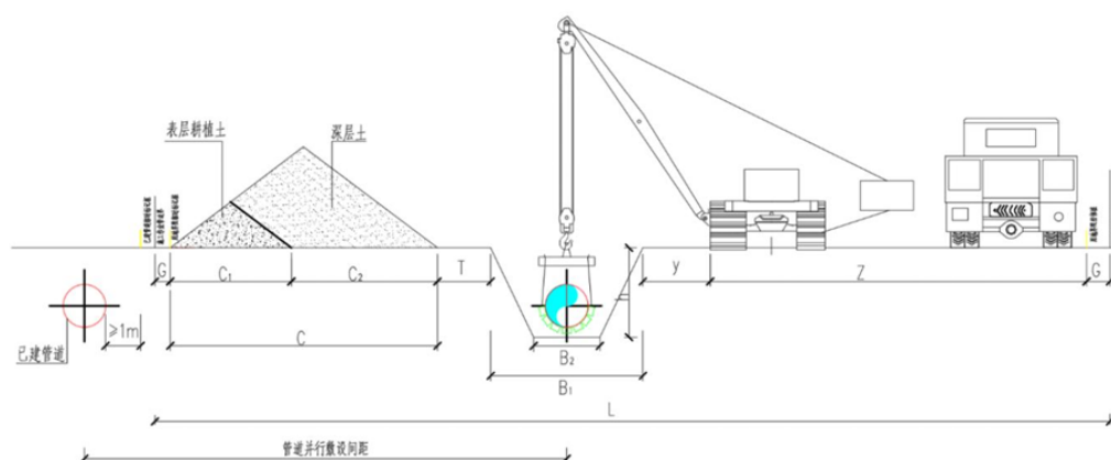
图 2.4-4 一般地段施工作业带
