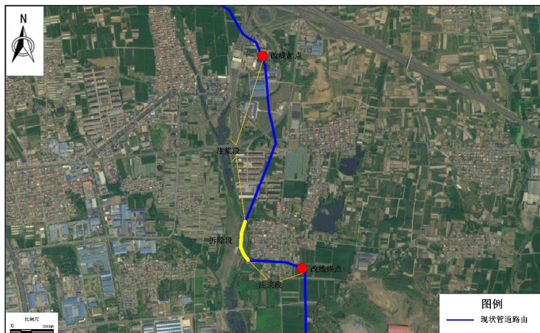
图 2.4-6 旧管道处置方案图（除穿越河流处拆除，其余旧管道均注浆处置）
