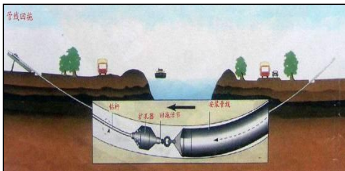
图 2.10-7 定向钻穿越施工管线回拖过程断面示意图
