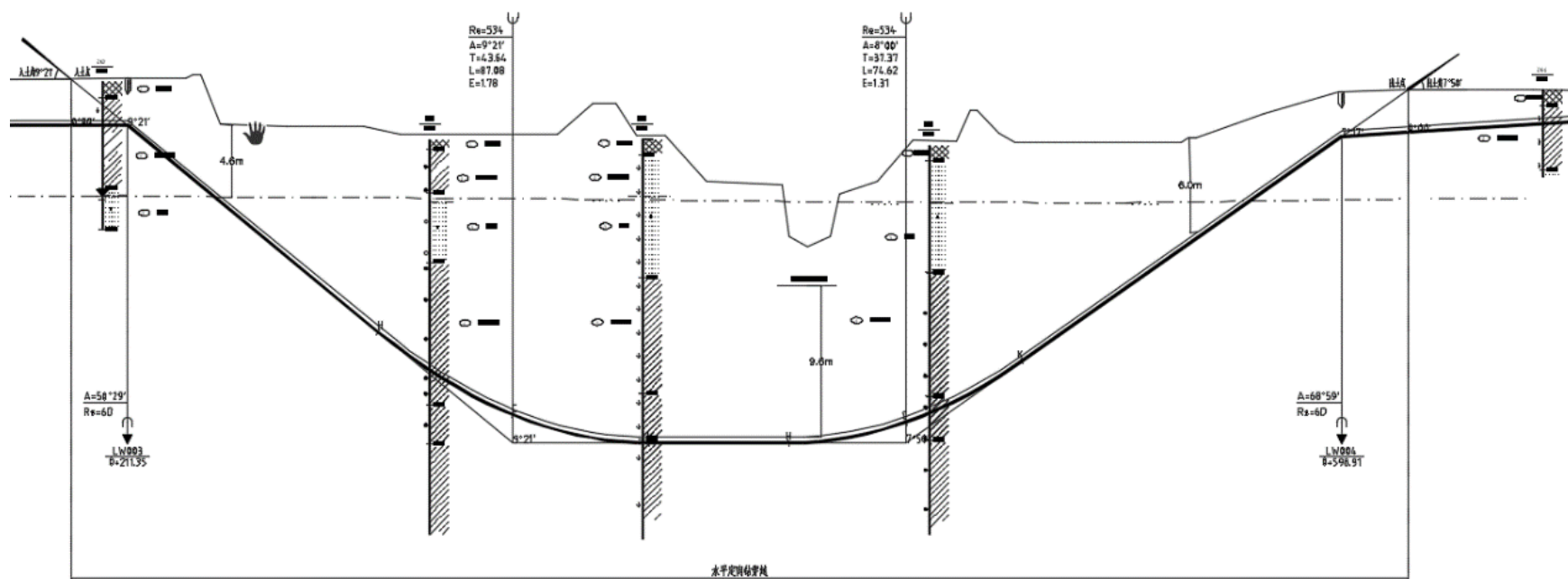
图 2.10-10 定向钻穿越断面示意图
