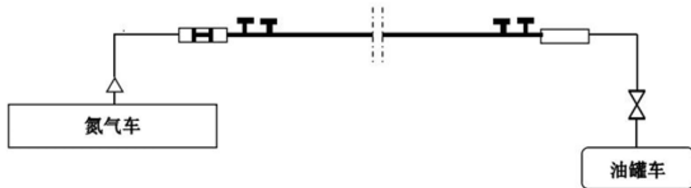
图 2.10-14 油品回收系统图
