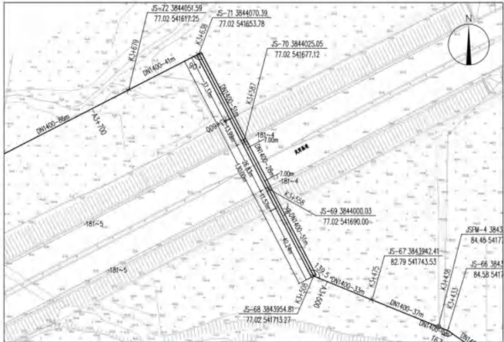
图 2.4-37 项目顶管穿越平面布置图
