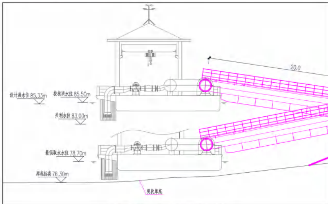
图 2.4-20 浮船泵站设计图
