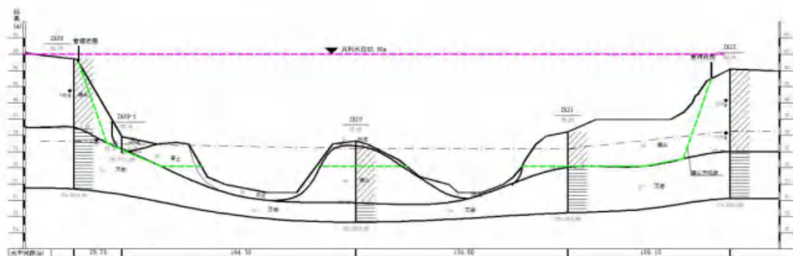
图 2.4-16 3-3'清淤断面图
