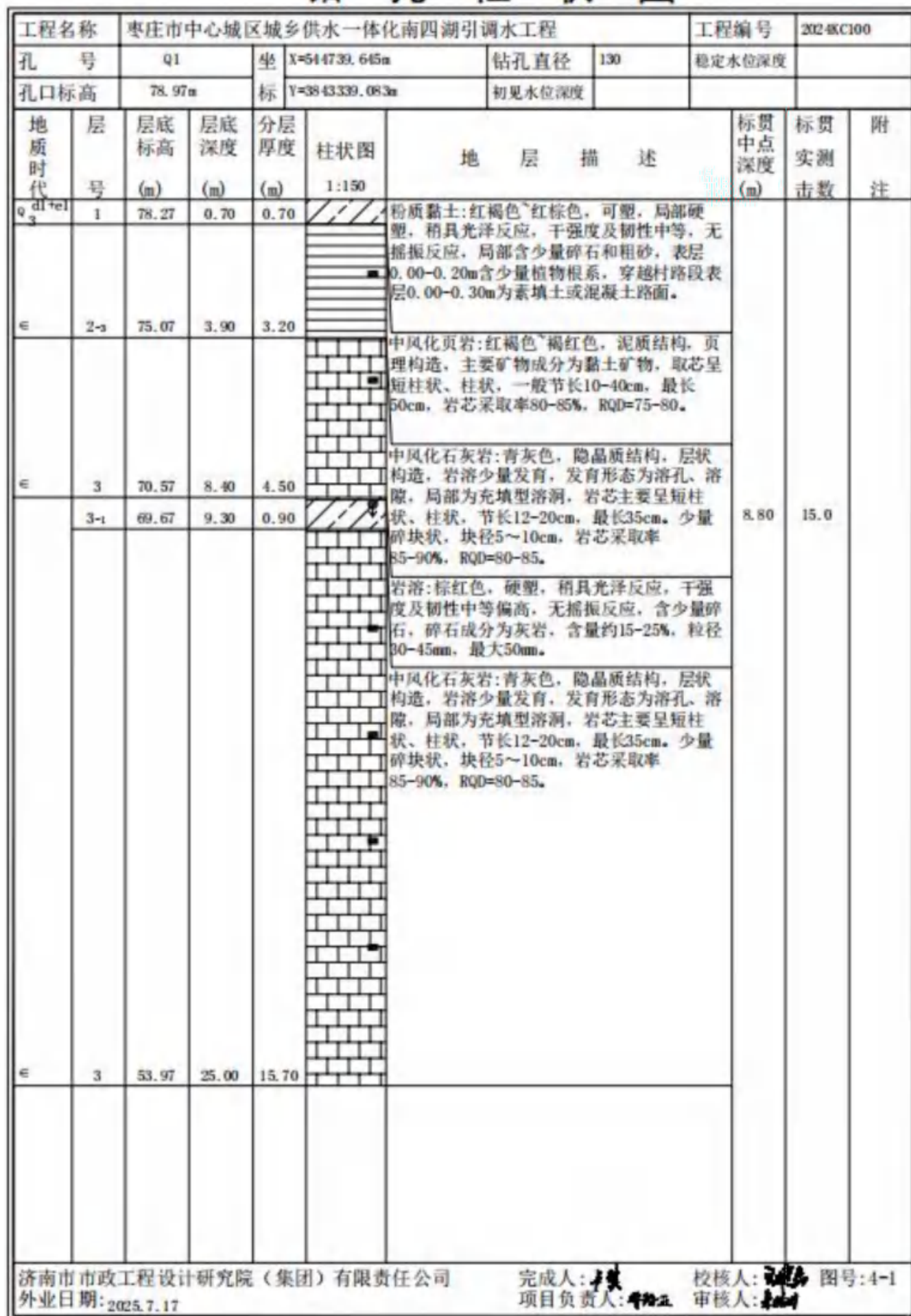
图 4.3-1 钻孔柱状图
