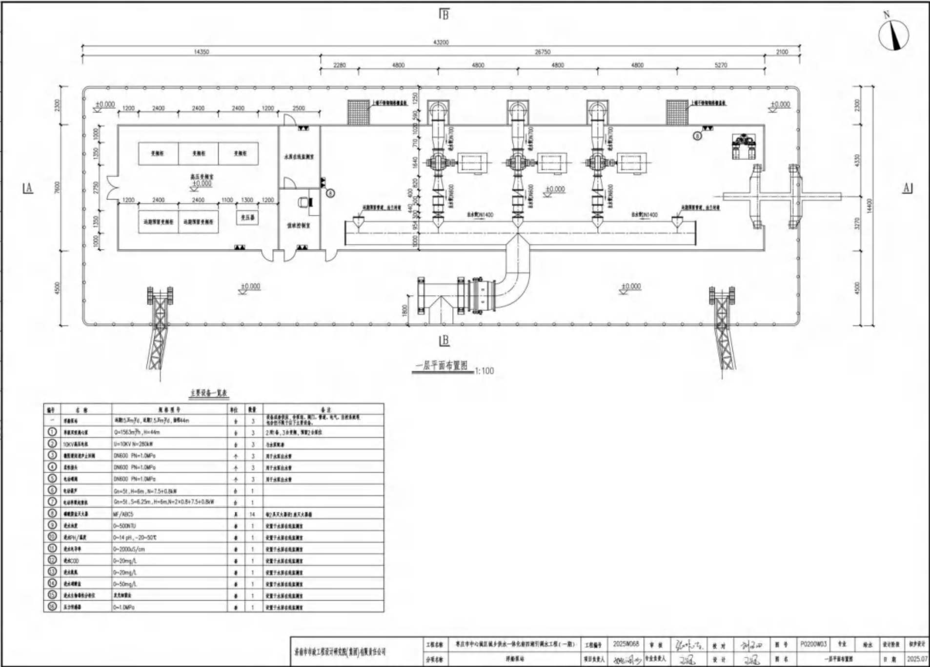
图 2.4-9（2） 本项目浮船泵站平面布置图（泵站一层）
