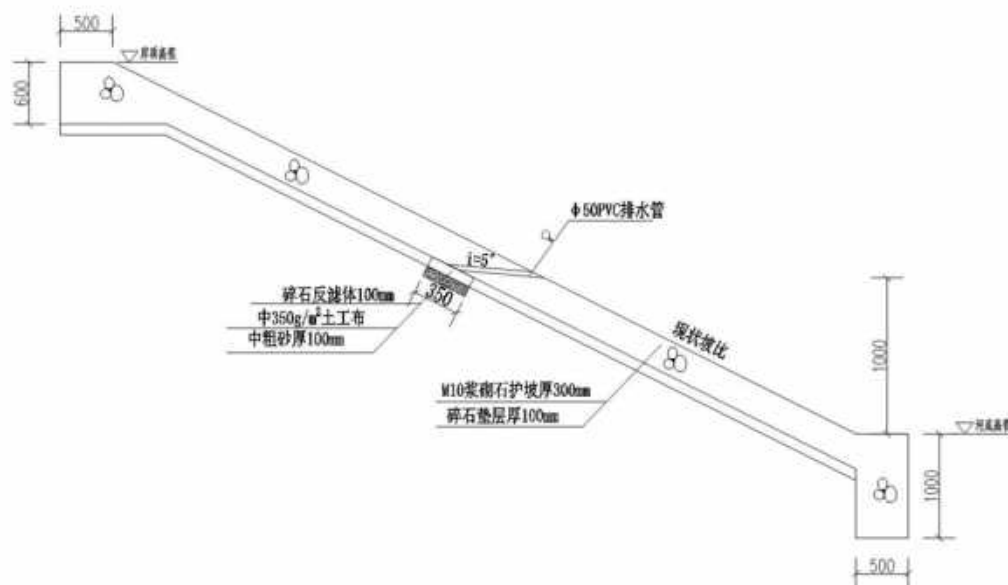
图 2.4-23 护岸设计标准断面图
