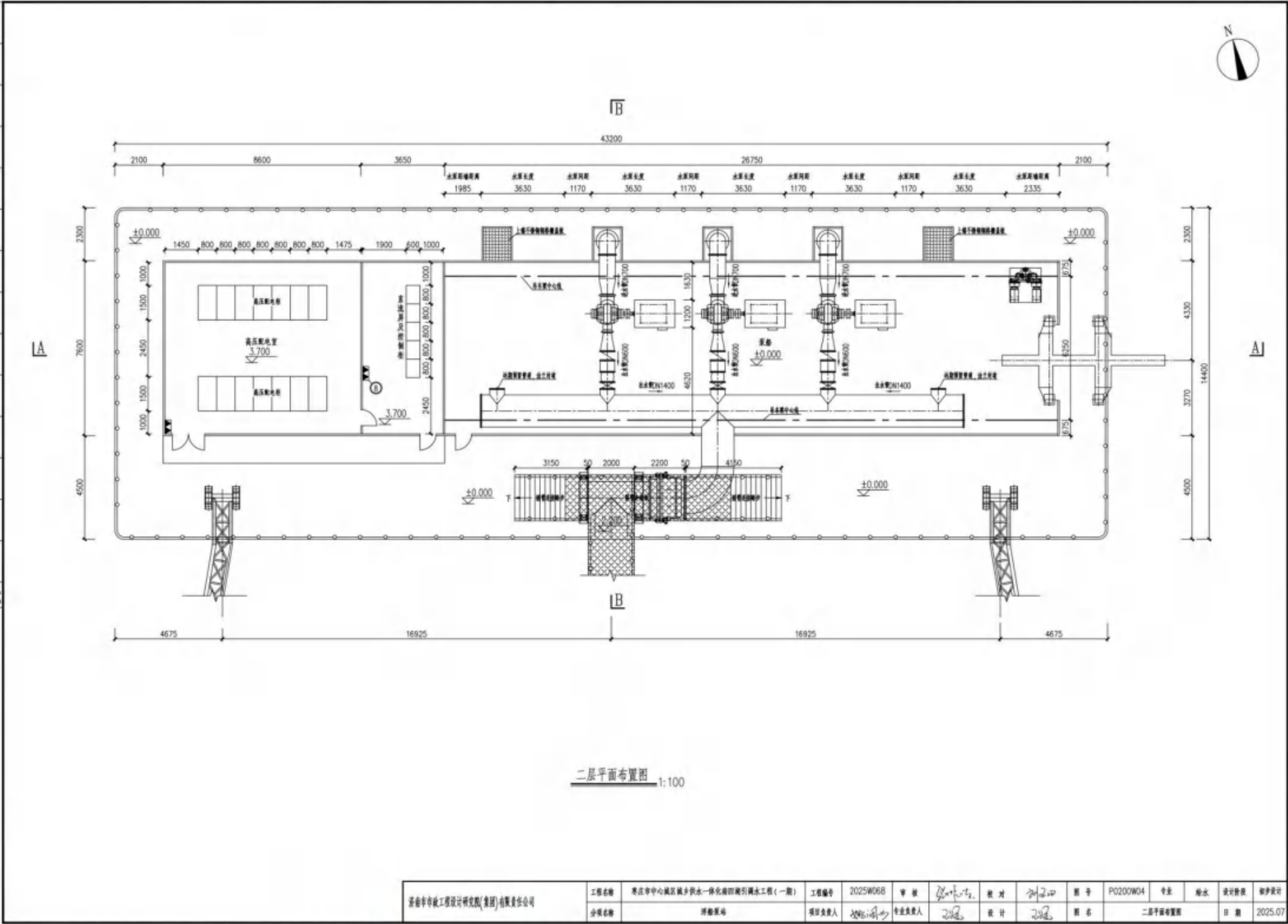
图 2.4-9 (3) 本项目浮船泵站平面布置图 (泵站二层)
