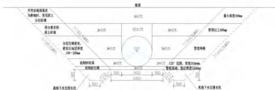
图 2.4-21 管道沟开挖及回填大样图
