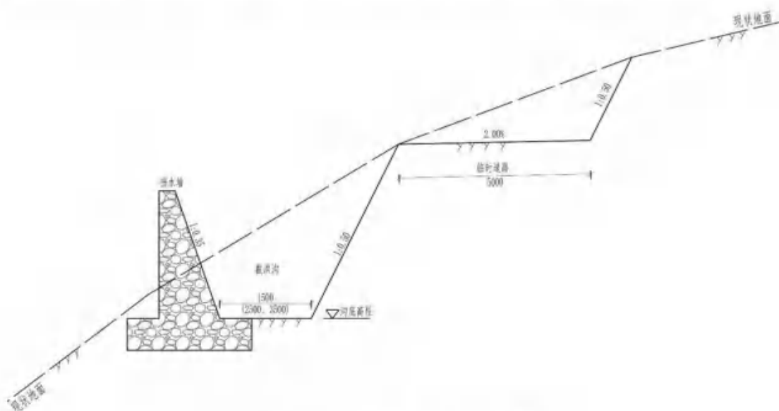
图 6.6-1 截渗沟剖面示意图
